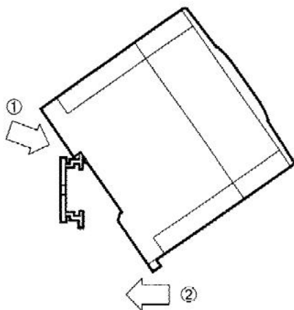
当将 FX2N-2LC插接到 DIN槽上时
