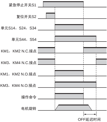
时序图
