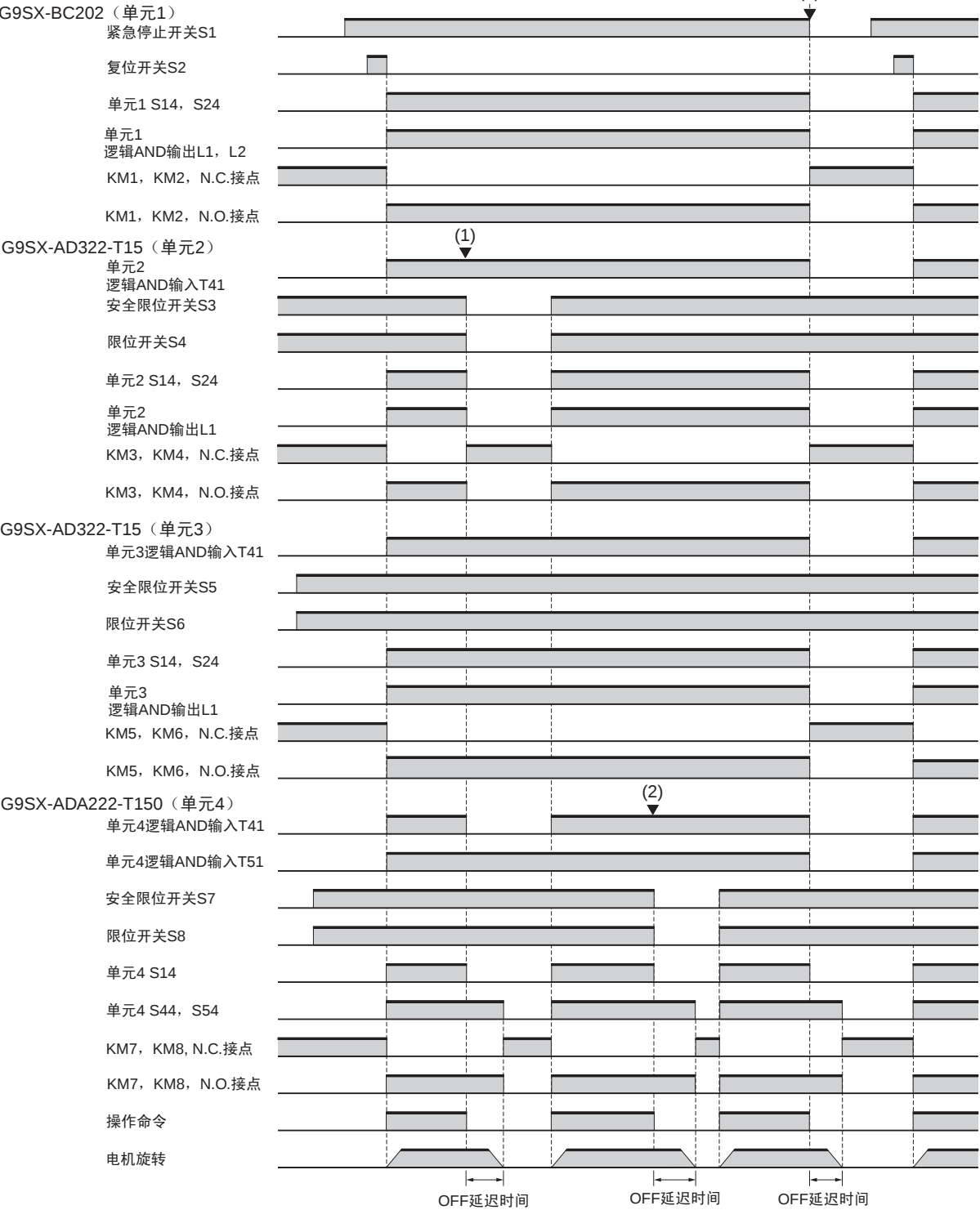
时序图
