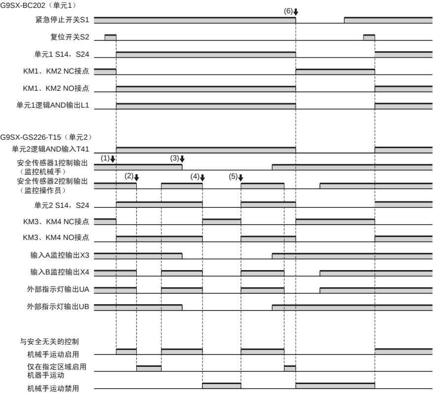
时序图1
