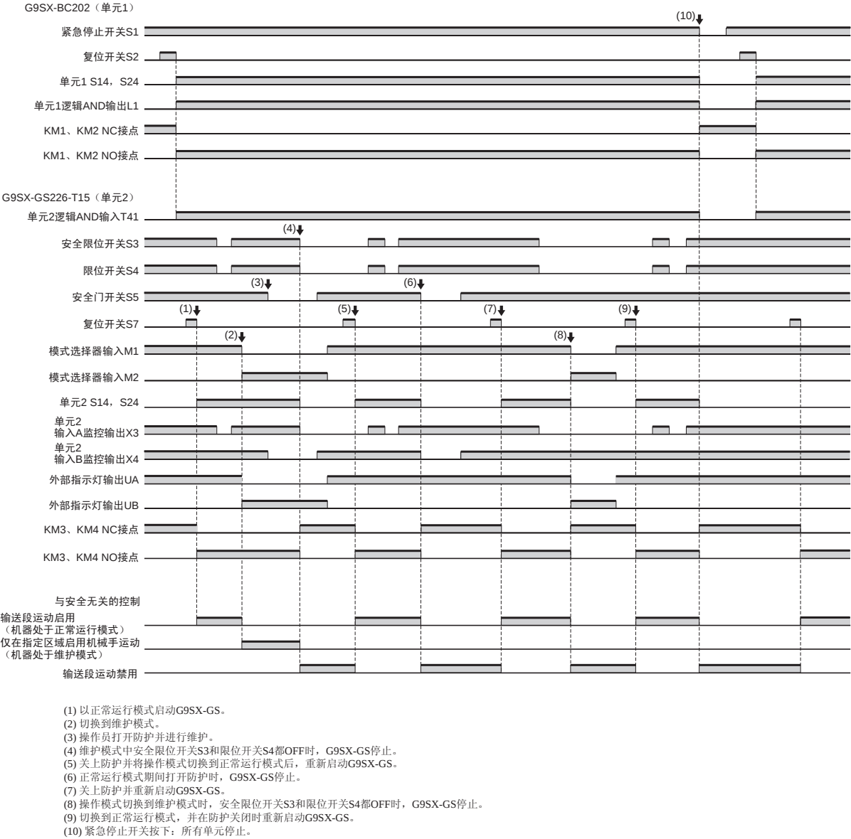
时序图2
