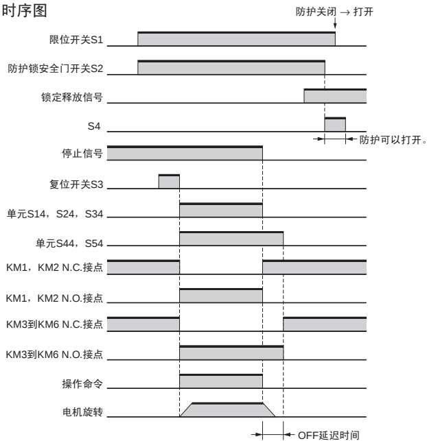
时序图
