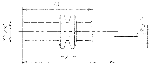
E2EL-X2□-L 2M, E2EL-X4□-DL 2M, E2EL-X4□-DSL 2M
