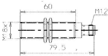
E2EL-X5□-M1L, E2EL-X8□-DM1L, E2EL-X8□-DM1SL
