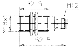
E2EL-X5□-M1, E2EL-X8□-DM1, E2EL-X8□-DM1S
