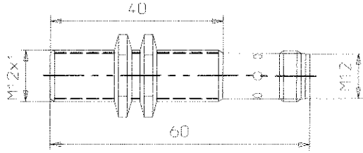
E2EL-X2□-M1L, E2EL-X4□-DM1L, E2EL-X4□-DM1SL
