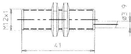
E2EL-X2□-L 2M, E2EL-X4□-DL 2M, E2EL-X4□-DSL 2M
