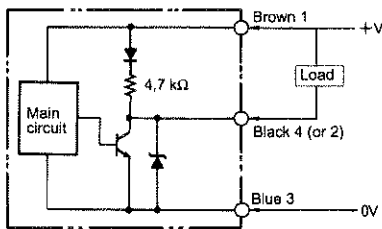
E2EL-X□E□ NPN Output
